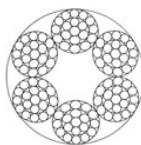
6 x 19 + FE
