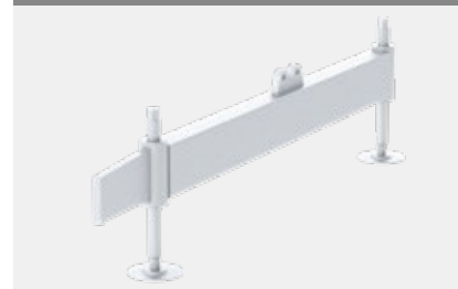
LONG OUTRIGGER M12 231003 10.1 kg
